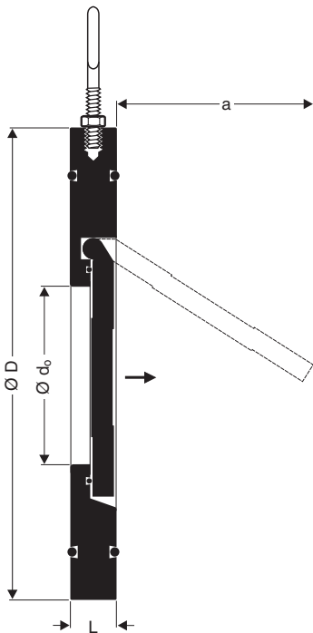
WB 26, WB 26A, WB 24 S DN 50 bis 300
